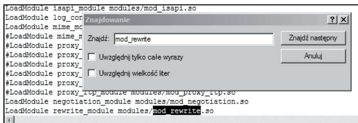
Rysunek 7.6. Wyszukiwanie modułu mod_rewrite
