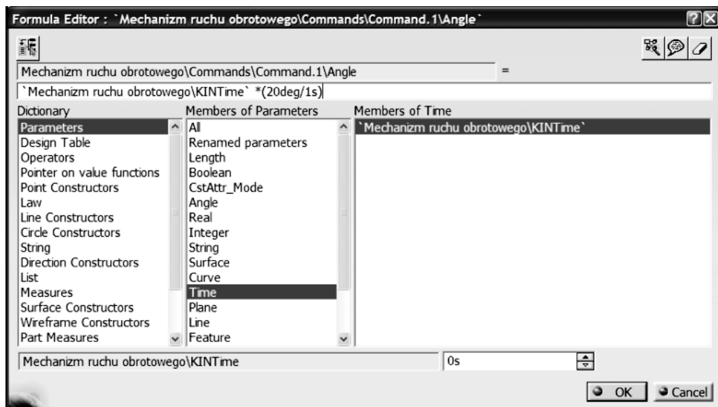
Rysunek 5.33. Zapis formuły sterującej ruchem obrotowym — okno Formula Editor
