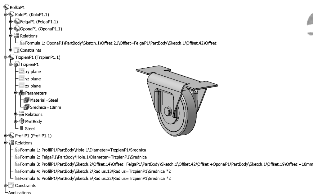
Rysunek 4.26. Złożenie RolkaP1 cechuje się prawidłowym umiejscowieniem relacji w strukturze drzewa, co skutkuje brakiem konieczności stosowania parametrów zewnętrznych
