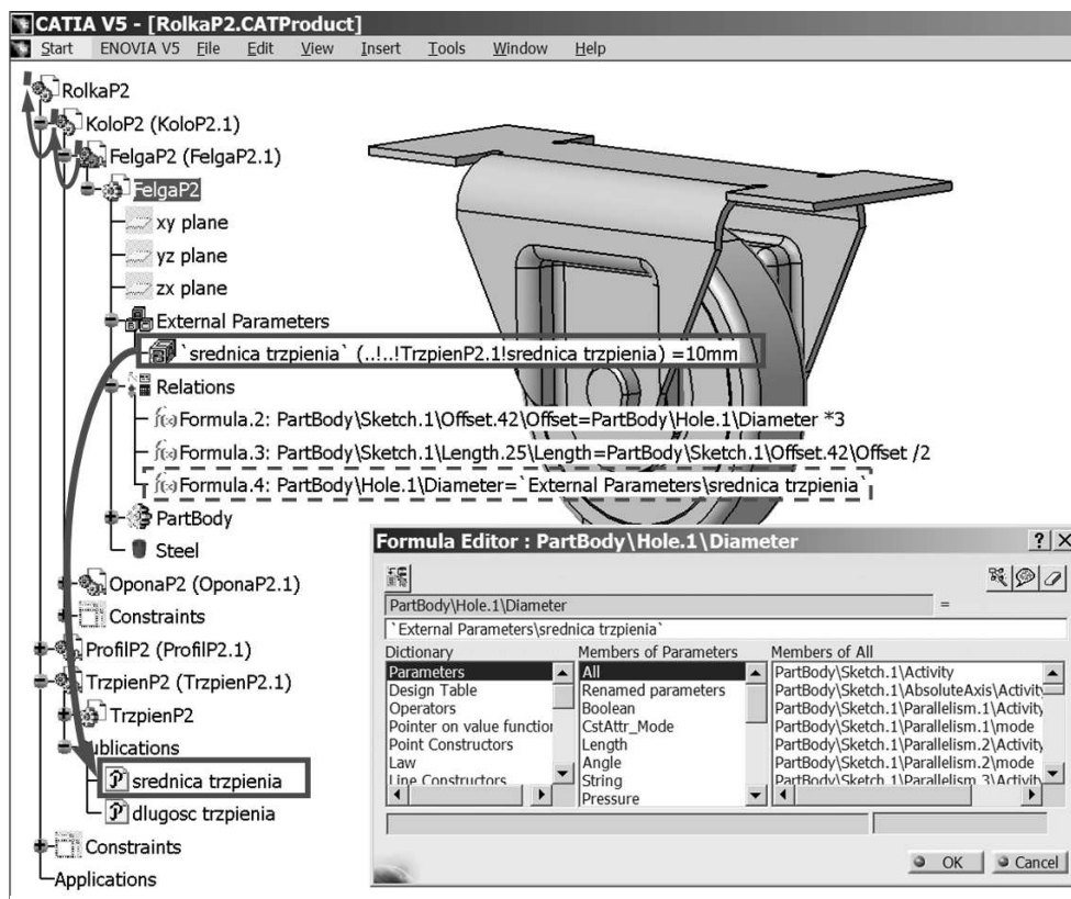
Rysunek 4.19. Wykorzystanie parametru zewnętrznego z publikowanego parametru z uwzględnieniem kontekstu zaznaczone jest znakami ...!..!
