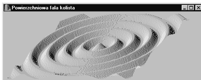
Rysunek 3.3. Powierzchniowa fala kolista, której formuła zawiera dość istotny błąd — amplituda nie maleje wraz z odległością
