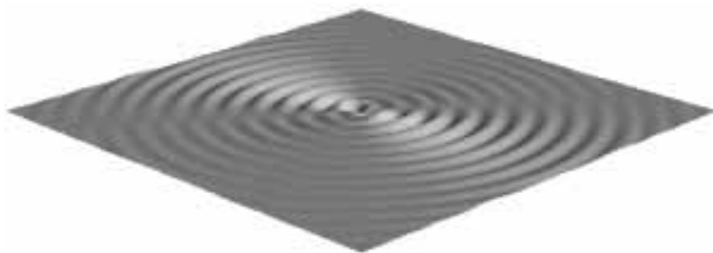
Rysunek 3.8. Fala o długości 4 cm jest wzbudzana w dwóch miejscach oddległych od siebie o 4 cm. Słabo widoczne są obszary interferencyjnych wzmocnień i osłabień — odległość źródeł jest zbyt mała w porównaniu z długością fali
