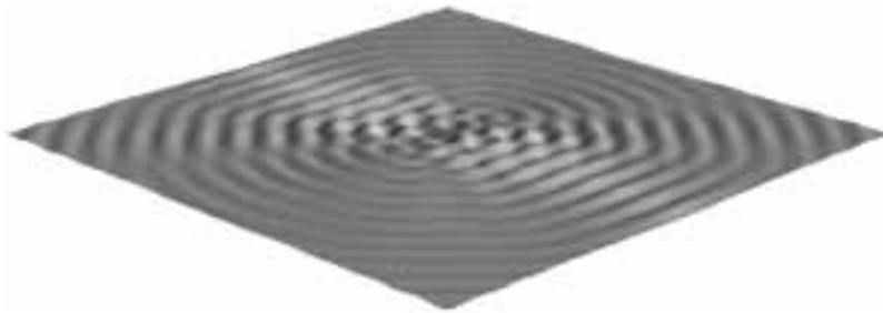
Rysunek 3.12. Obraz powierzchni wody pobudzonej do harmonicznego drgań w pięciu równoodległych punktach
