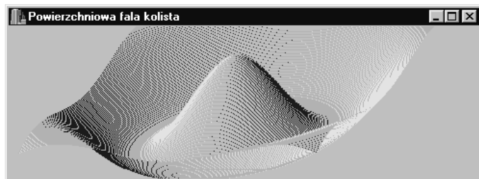
Rysunek 3.4. Realistyczny obraz fali powierzchniowej musi zawierać czynnik tłumiący amplitudę wraz ze wzrostem odległości — im dalej, tym mniejsza fala. Oto wykres funkcji F(x, y) = 50 * \exp(-r / 100) * \cos(r) . Funkcja ta maleje wraz z odległością
