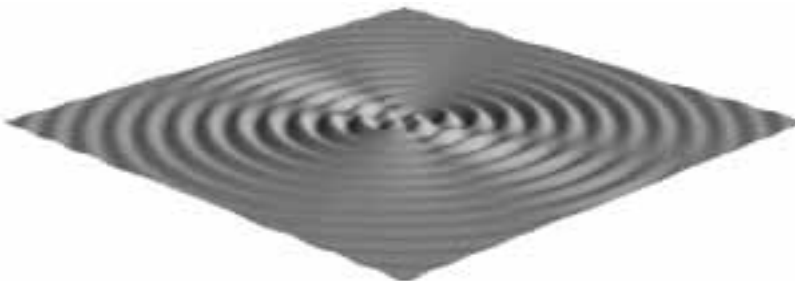
Rysunek 3.9. Takie same fale, ale wzbudzone w miejscach oddległych od siebie o 10 cm. Teraz obszary oddziaływań interferencyjnych są znacznie lepiej widoczne
