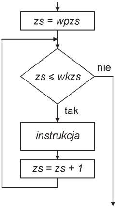
Rysunek 4.1. Pętla ze zmienną sterującą — odliczanie w górę
