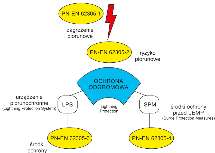
Rys. 1.1. Schemat wzajemnej zależności aktualnych norm odgromowych
