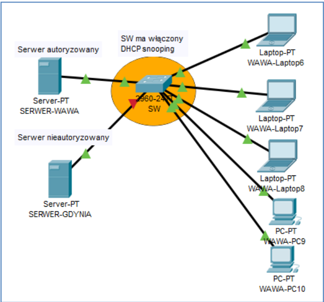
Rysunek 9.7 Topologia sieci z użyciem DHCP snooping.
