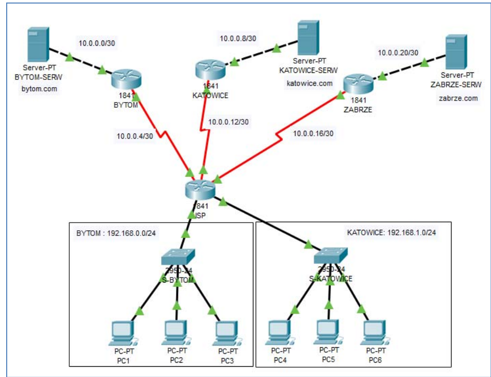
Rysunek 9.3. Topologia logiczna sieci.
