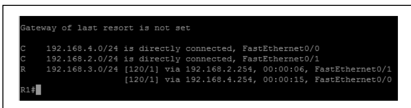
Rysunek 5.24. Tablica trasowania routera R1
