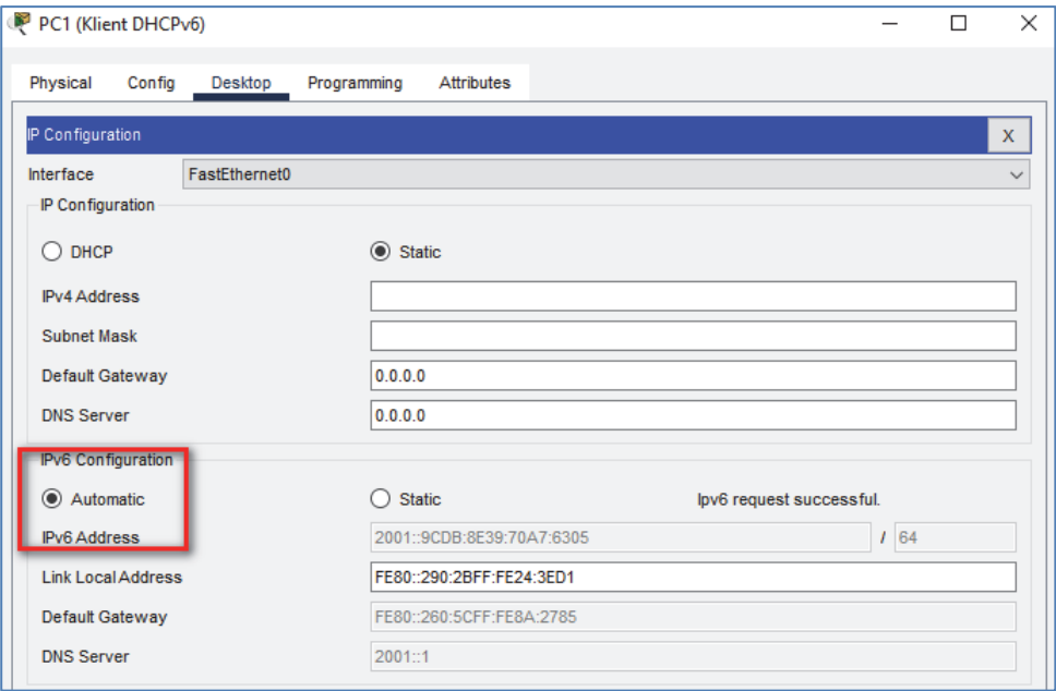
Rysunek 3.37 Konfiguracja IPV6 w PC1
