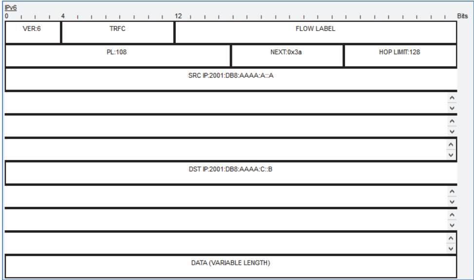
Rysunek 3.2. Przykładowy pakiet IPV6 w programie Packet Tracer 8.1.1
