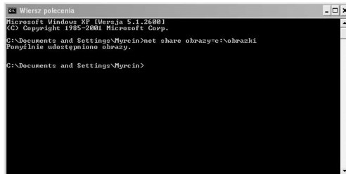
Rysunek 5.23. Polecenie net share jest bardzo przydatne, gdy musisz szybko udostępnić wiele folderów jednocześnie. Możesz wtedy stworzyć skrypt udostępniający foldery
