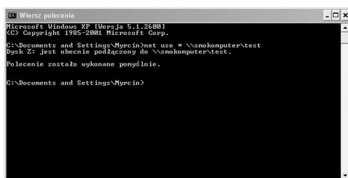
Rysunek 5.22. Możesz używać polecenia net use również w skryptach użytkownika
