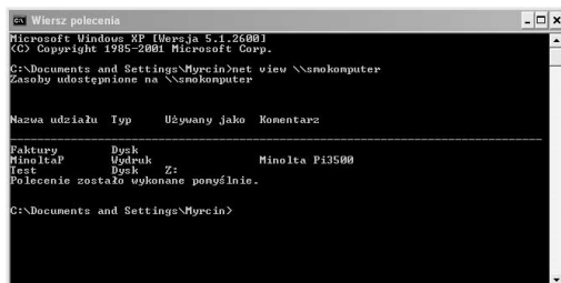
Rysunek 5.21. Polecenie net view pozwala przeglądać zasoby komputera zdalnego
