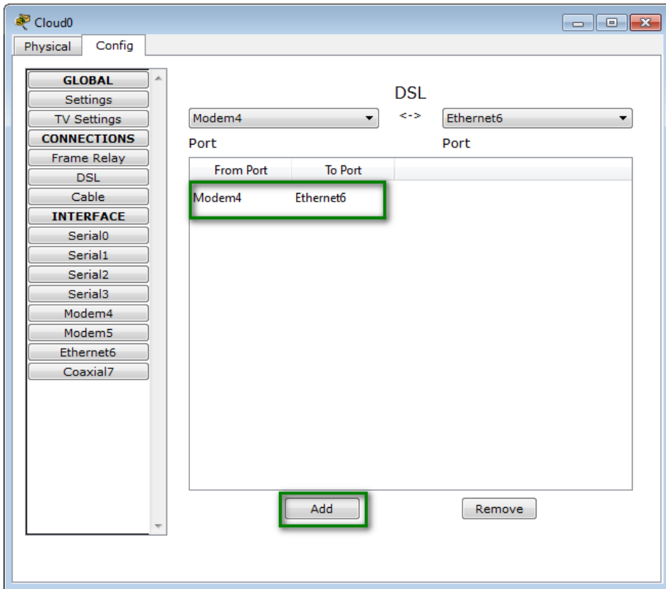
Rysunek 5.15 Konfigurowanie DSL (Modem4 – Ethernet6)
