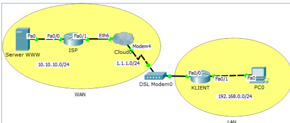
Rysunek 5.9 Topologia sieci
