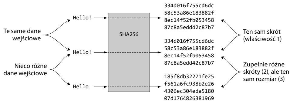
Rysunek 2.11. Kryptograficzna funkcja skrótu SHA256 w działaniu. Dla danych wejściowych „Hello!” daje za każdym razem ten sam skrót, ale nawet niewielka zmiana (na „Hello”) daje zupełnie inny skrót
