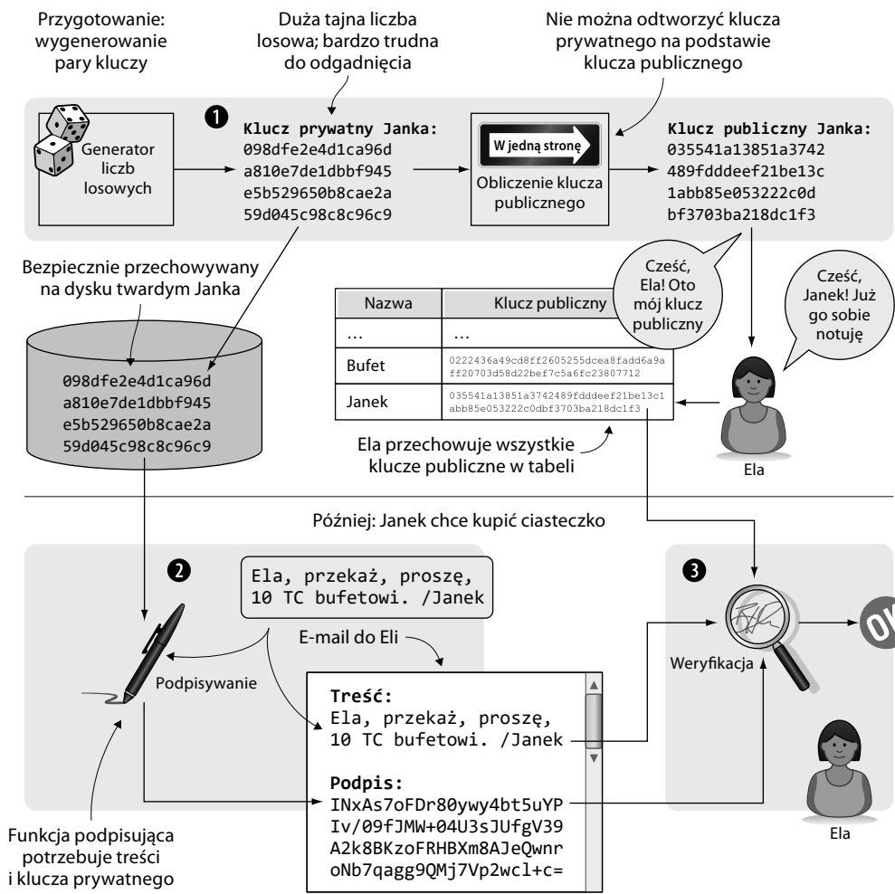
Rysunek 2.15. Proces składania podpisu cyfrowego. ❶ Janek tworzy parę kluczy i przekazuje klucz publiczny Eli. ❷ Janek podpisuje wiadomość za pomocą swojego klucza prywatnego. ❸ Ela sprawdza, czy wiadomość została podpisana kluczem prywatnym powiązanim z kluczem publicznym, który otrzymała od Janka
