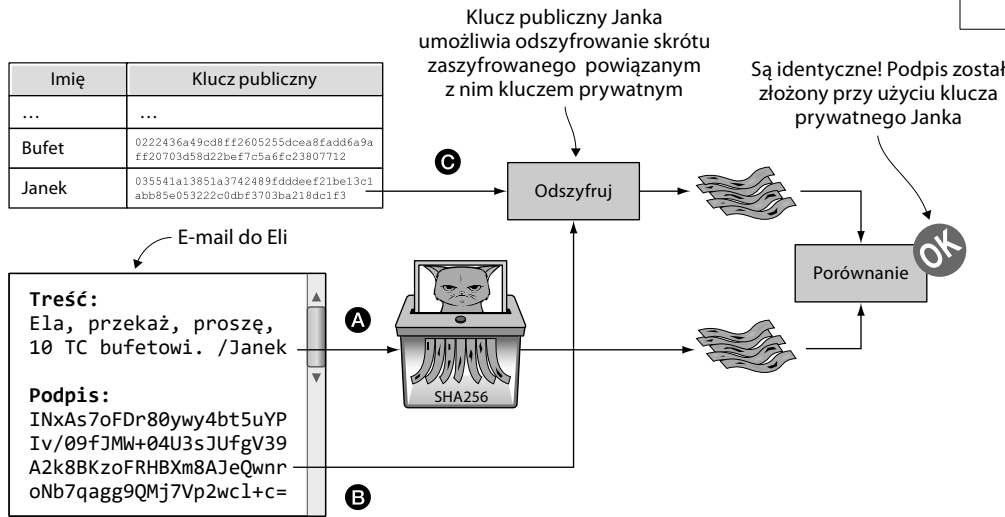
Rysunek 2.20. Za pomocą podpisu (B) i klucza publicznego (C) Janka Ela sprawdza, czy treść wiadomości (A) została podpisana kluczem prywatnym Janka
