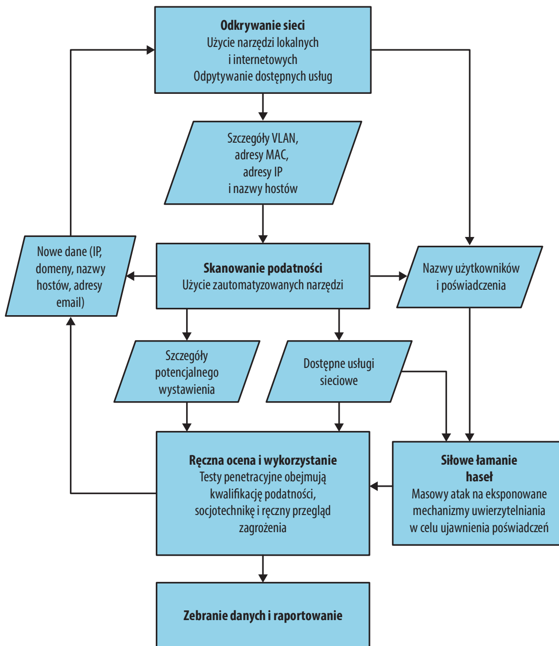
Rysunek 2-3 Podjęcie iteracyjne do odkrywania i testów
