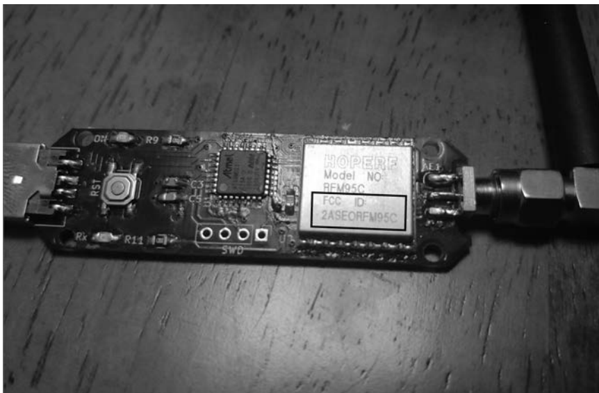
Rysunek 3.2. Identyfikator FCC układu RFM95C zastosowanego w urządzeniu USB CatWAN, które wykorzystamy w rozdziale 13. do hakowania sieci LoRa
