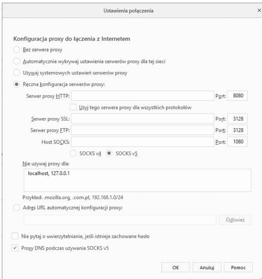
Rysunek 2.12. Okno ustawień proxy przeglądarki Firefox
