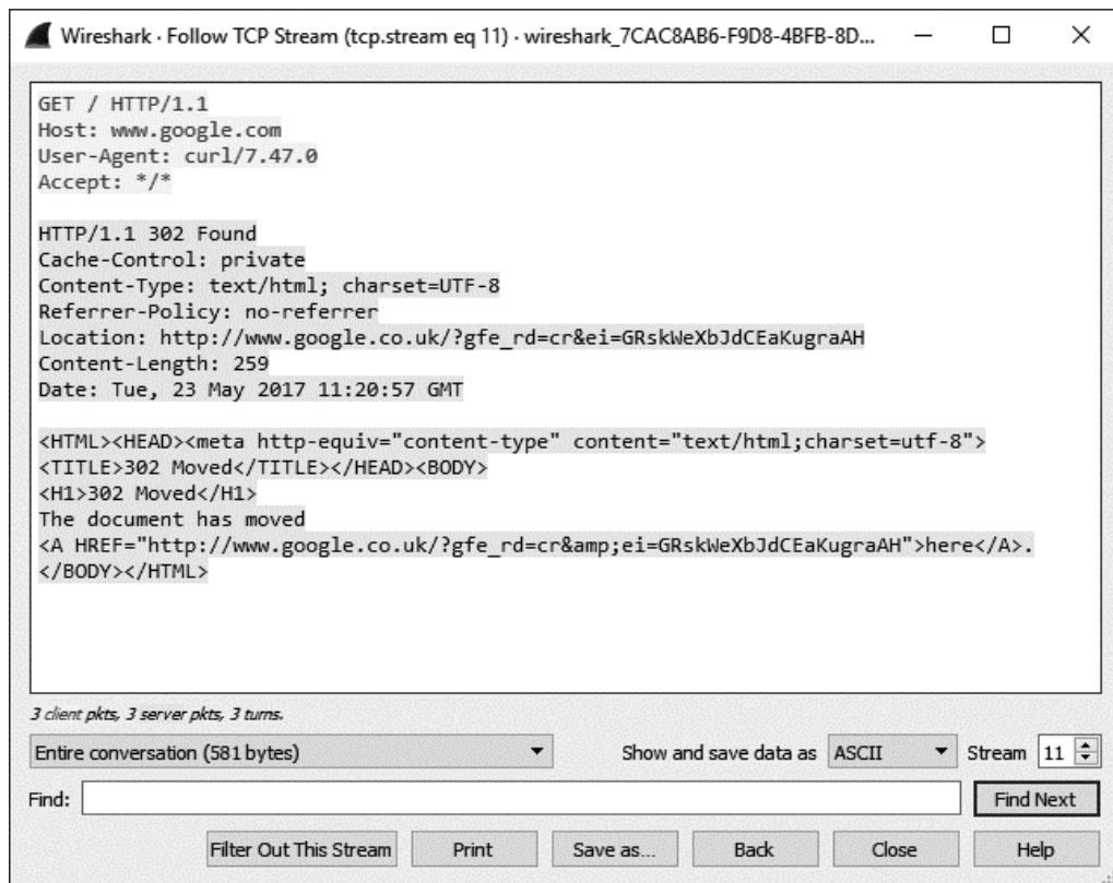
Rysunek 2.3. Czytelna prezentacja strumienia TCP w oknie programu Wireshark
