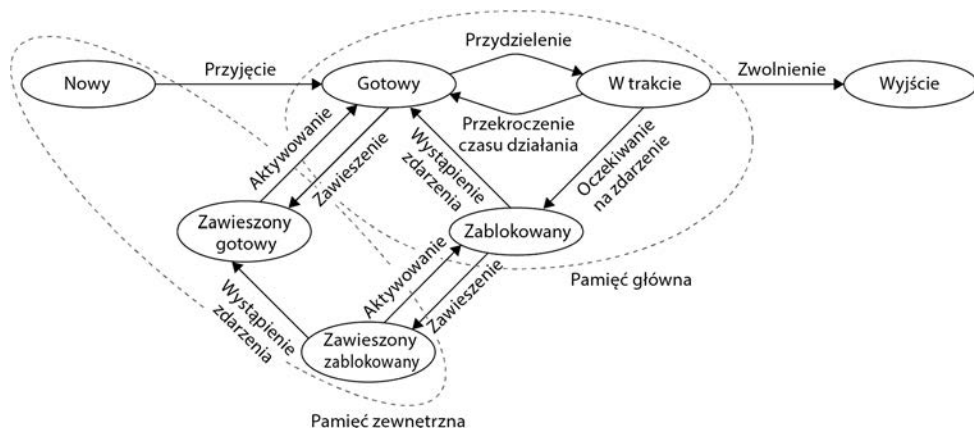
Rysunek 3.3. Stany procesów w systemach operacyjnych
