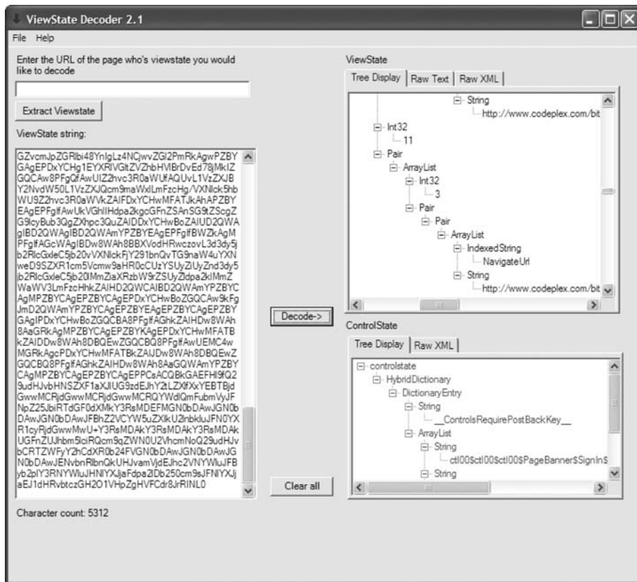
Rysunek 4.4. Dekodowanie danych przesyłanych za pomocą mechanizmu ViewState języka ASP.NET
