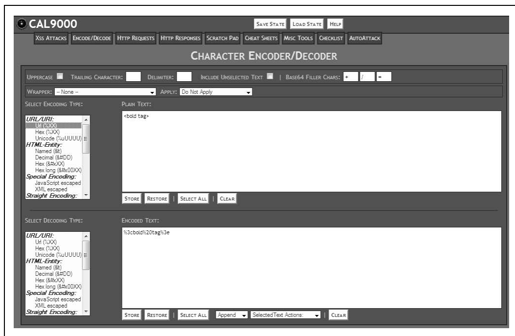
Rysunek 4.2. Kodowanie URL za pomocą narzędzia CAL9000
