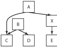
(d) Rozdzielenie B od A. Zwróć uwagę, że w B nadal mogą być czytelnicy. Wszystkie procesy-czytelnicy w B będą widziały starą wersję drzewa, natomiast wszystkie procesy-czytelnicy w A będą widziały nową wersję
