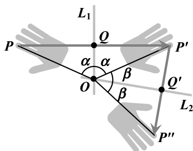
Rys. 1.10. Złożenie dwóch odbić
