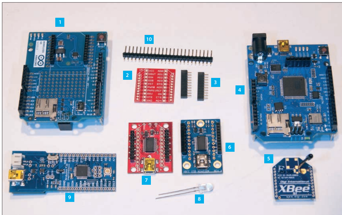
Rysunek 6.1. Nowe części w tym rozdziale: 1. Tarcza bezprzewodowa Arduino 2. Płytki stykowe Spark Fun XBee 3. Gniazda do listew kołkowych 2 mm 4. Tarcza Arduino Wi-Fi 5. Moduł Digi XBee 802.15.4 OEM 6. Adapter Adafruit XBee na USB 7. Spark Fun XBee Explorer 8. Dioda podczerwień 9. Arduino Fio. Nie zapomnij o mnóstwie listew kołkowych do płyt z wyprowadzeniami dla układów scalonych
