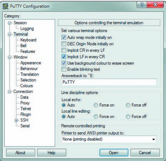
Rysunek 6.11. Menu Terminal Configuration w PuTTY. Aby użyć PuTTY do konfiguracji radia Digi (XBee i innych), wybierz „Implicit LF in every CR”
