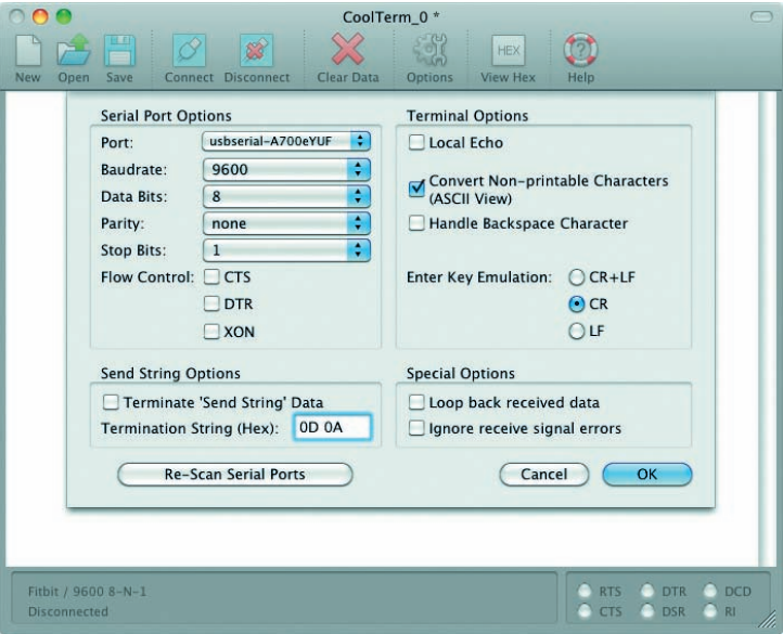
Rysunek 6.10. Menu opcji CoolTerm. Aby użyć CoolTerm do konfiguracji radioodbiorników Digi (XBee i innych), ustaw Enter Key Emulation na CR
