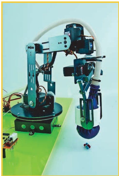
RYСУNEK 2.25. Robot Balloon Bot stworzony przez Steve’a Norrisa podnosi przedmioty za pomocą nietypowego mechanizmu opartego na zmielonych ziarnach kawy Zdjęcie: Steve Norris
