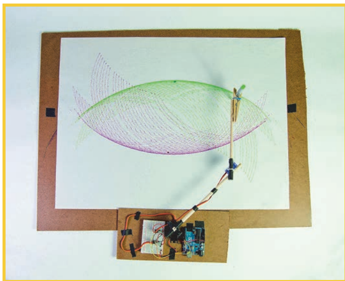
RYСУNEK 2.11. Robot Arc-O-Matic rysujący krzywe
