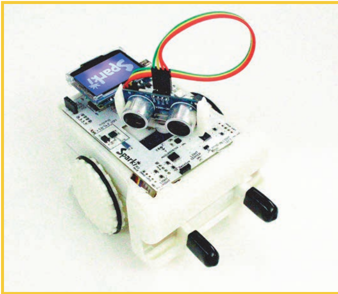
RYСУNEK 2.2. Robot Sparki jest gotowy do zaprogramowania od razu po wyjęciu z pudełka Zdjęcie: http://arcbotics.com/
