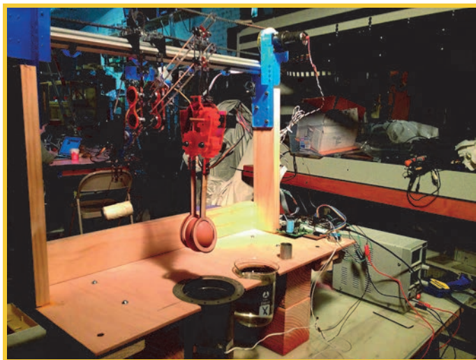
RYСУNEK 2.12. Robot Soft-Boiled Eggbot ugotuje za Ciebie śniadanie Zdjęcie: Trammell Hudson
