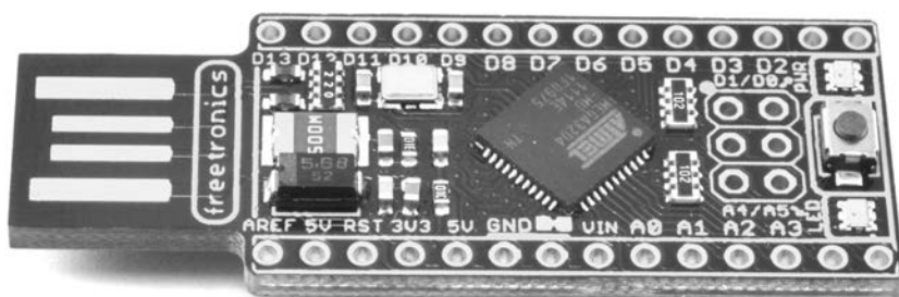
Rysunek 11.1. Płytki LeoStick
