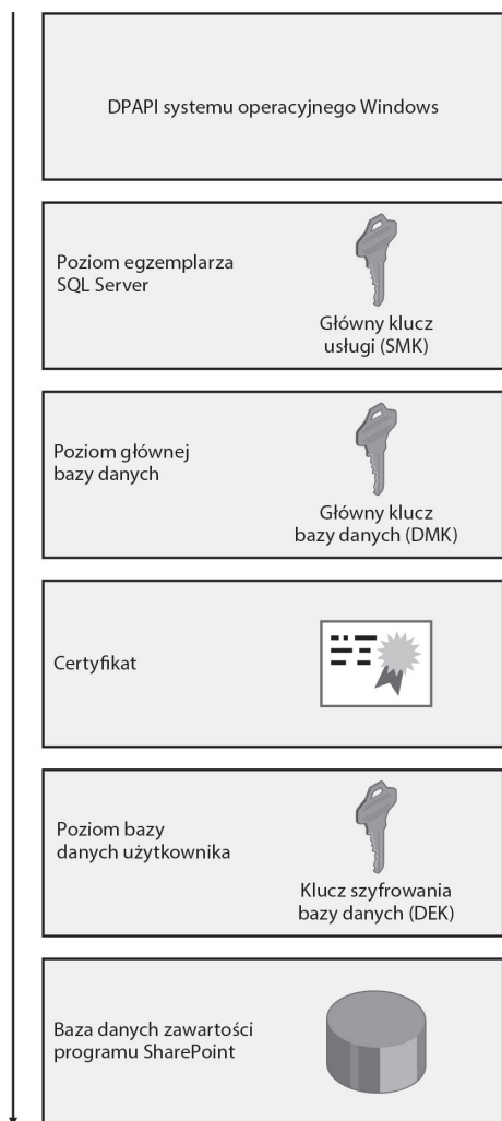
RYСУNEK 7.13. Architektura TDE
