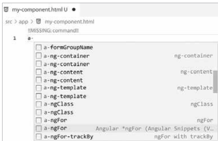
Rysunek 1.6. Fragment kodu z dyrektywą *ngFor
