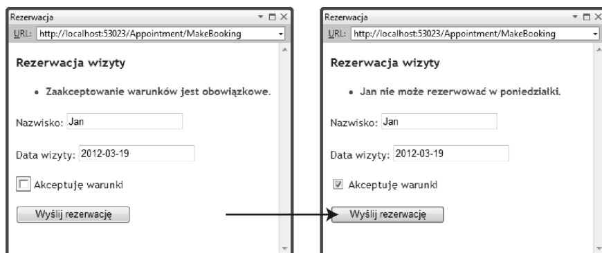
Rysunek 18.9. Stopniowe zgłaszanie problemów z wartościami wejściowymi
