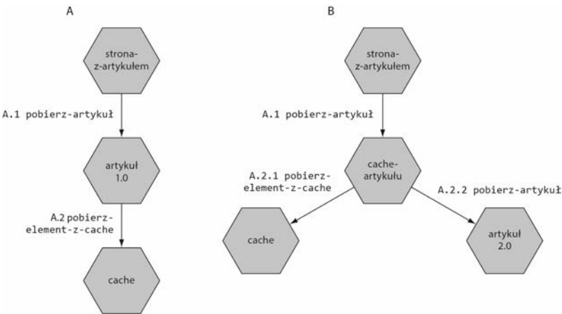
Rysunek 2.9. Rozszerzanie usługi artykuł bez modyfikacji
