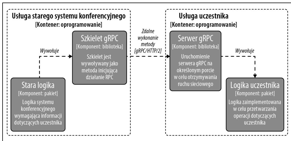
Rysunek 1.1. Przykładowy diagram C4 komponentu używającego standardu gRPC
