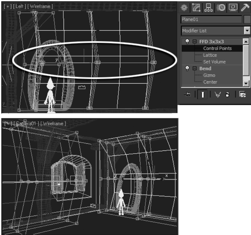
Rysunek 4.13. W wyniku przemieszczenia punktów kontrolnych modyfikatora FFD nałożonego na obiekt Plane01 (u góry) wyrzuszają się obie pajęczyny (u dołu)
