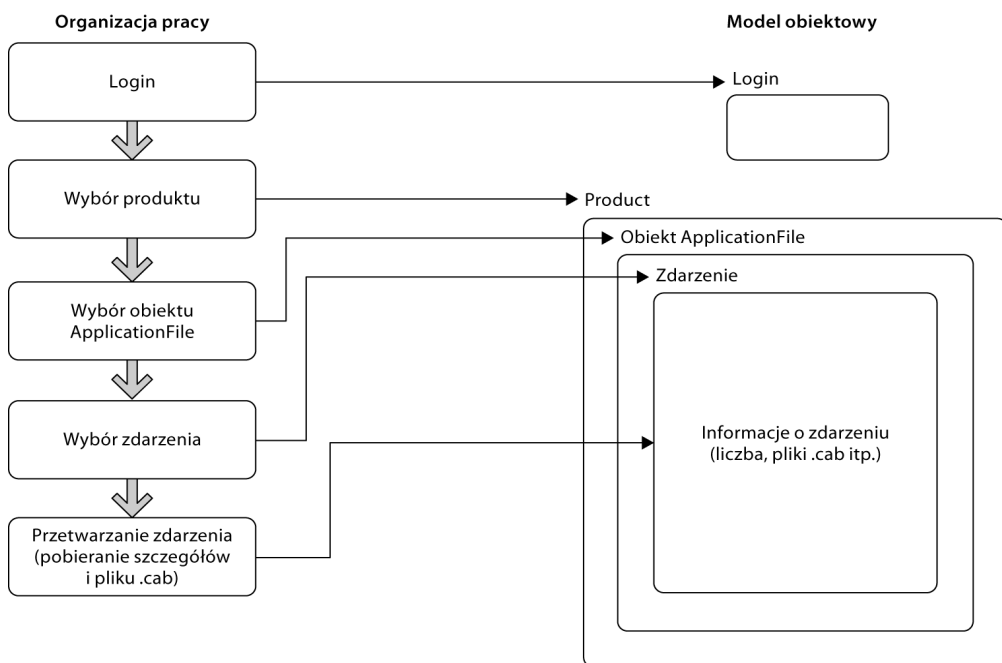
Rysunek 8.27. Schemat pracy WER i modelu klient-obiekt
