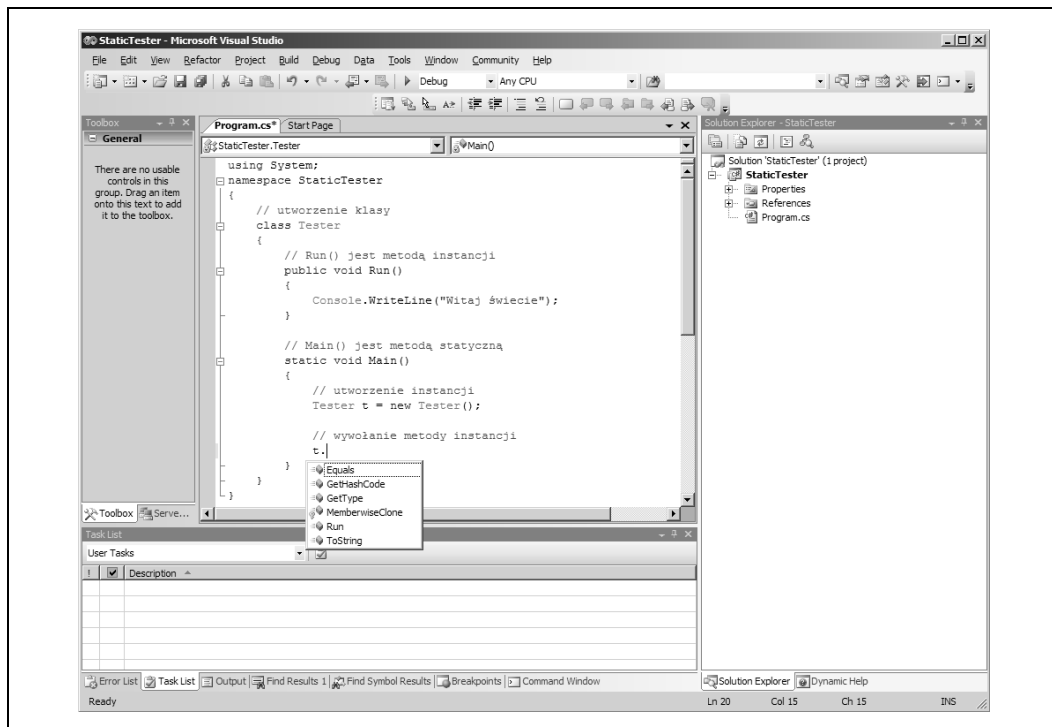
Rysunek 7.1. IntelliSense
